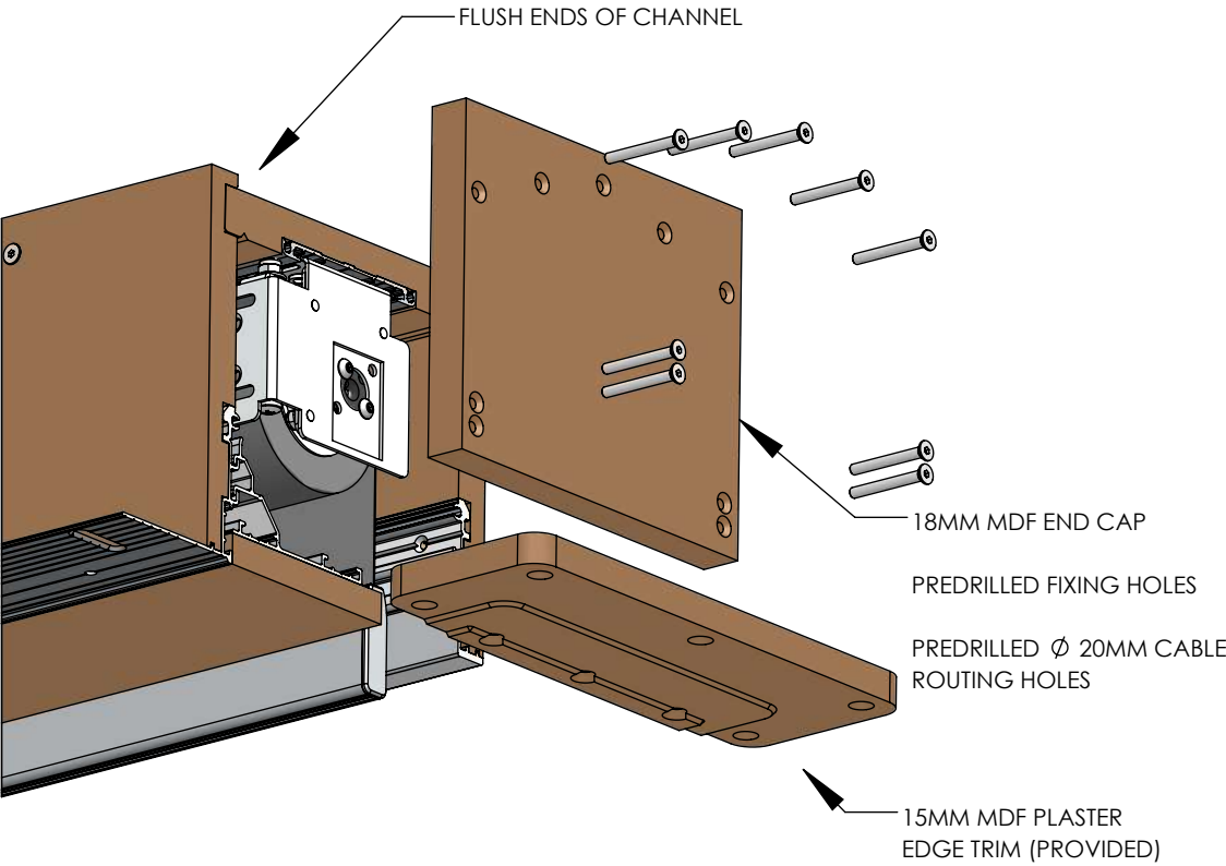
PLASTER EDGE END PLATE
