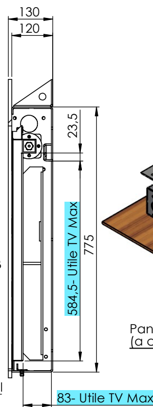
SEZIONE A-A
