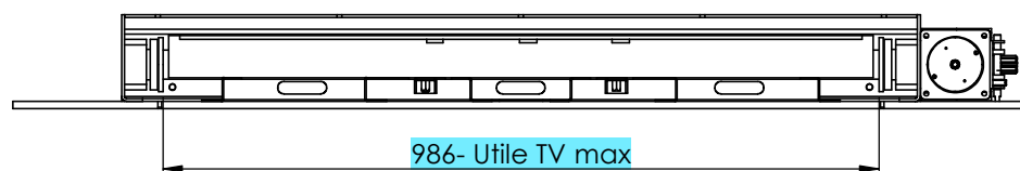
SEZIONE B-B
