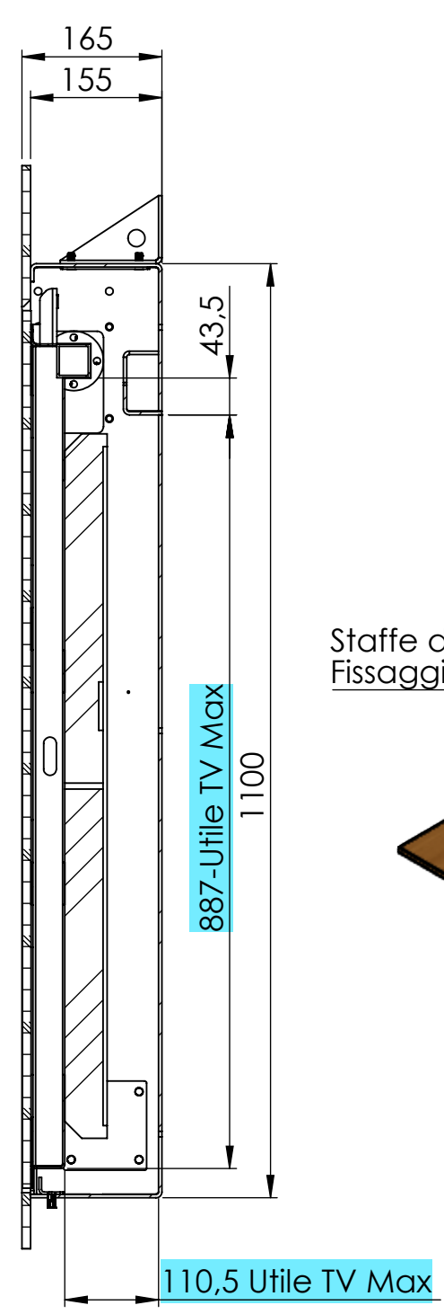
SEZIONE A-A
